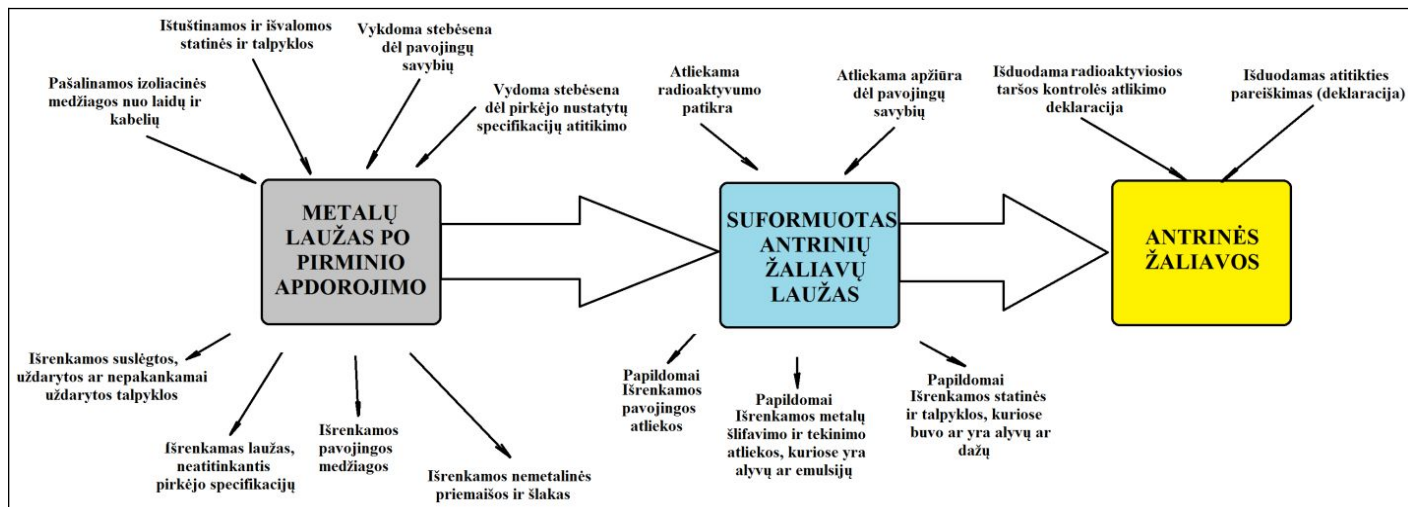
Metallų laužo perdirbimo į antrines žaliavas pagal Reglamento Nr. 333/2011 reikalavimus proceso schema
