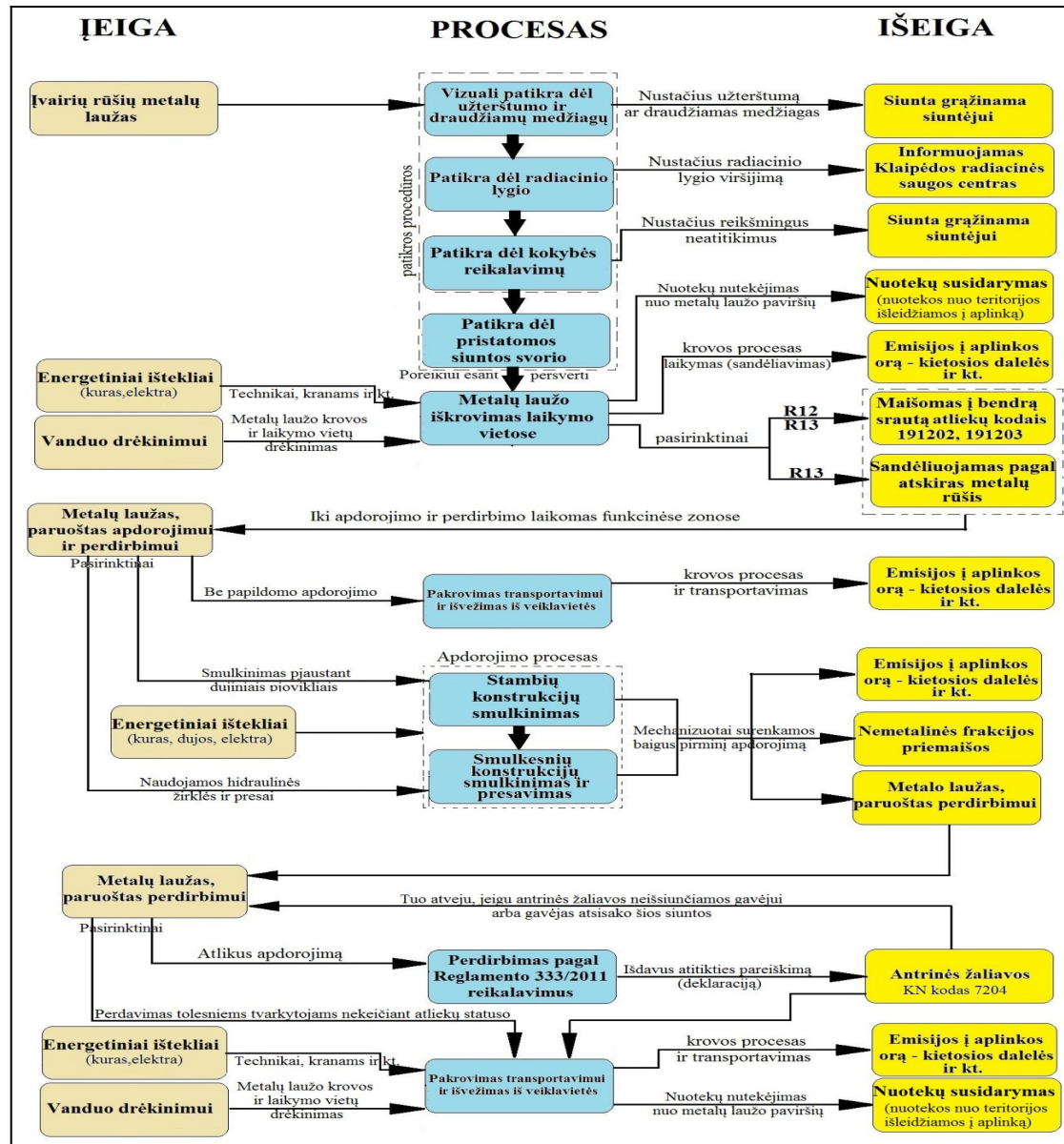
Netauriųjų metalų laužo ir atliekų tvarkymo technologinio proceso schema Nr. 3
